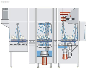
Schematischer Maschinenschnitt
